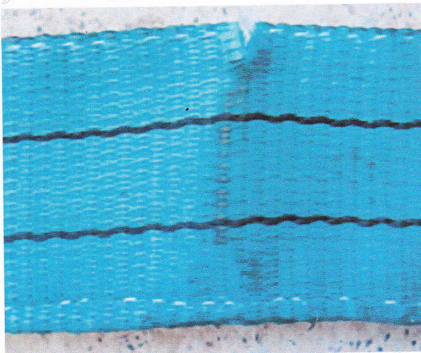
Bild 4-2: Unzulässiger Einschnitt an der Hebekante
