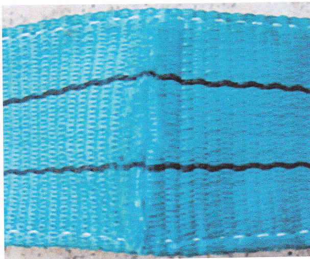
Bild 4-1: Unzulässiger Einschnitt an der Oberfläche
