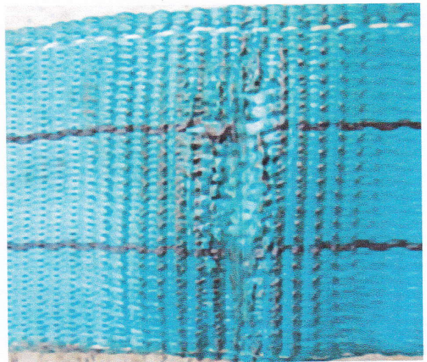
Bild 4-4: Durch heißen Span beschädigte Oberfläche
